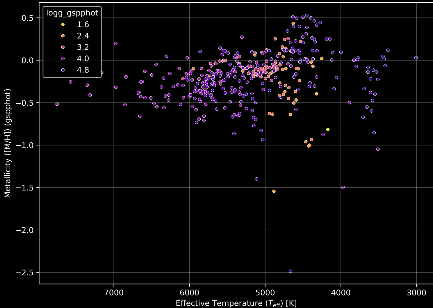
APOGEE DR17 Field: [120+30] Stellar Population Parameters (n= 393)
